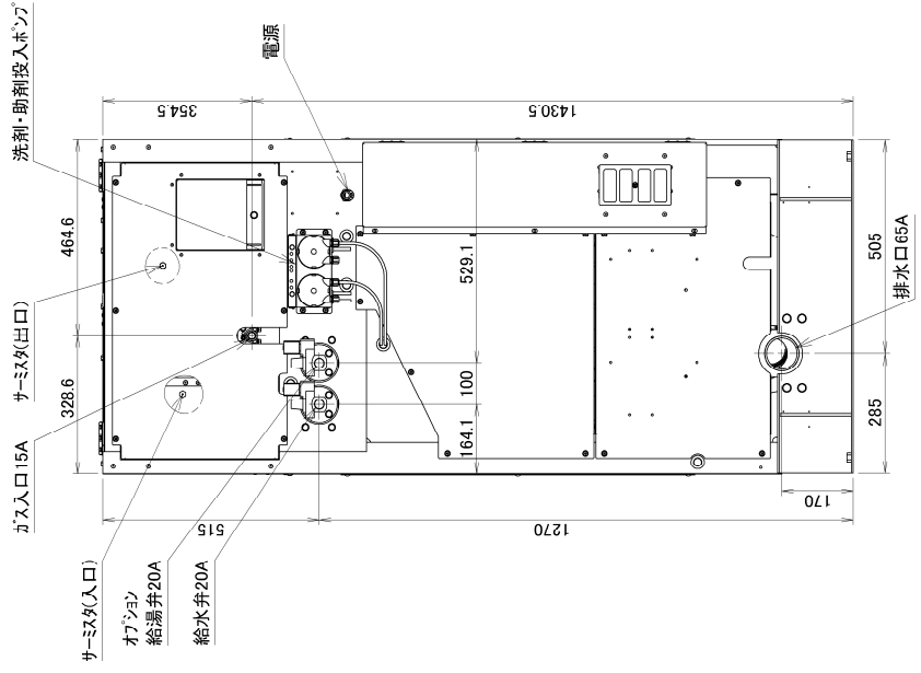
WD120CS外觀図
