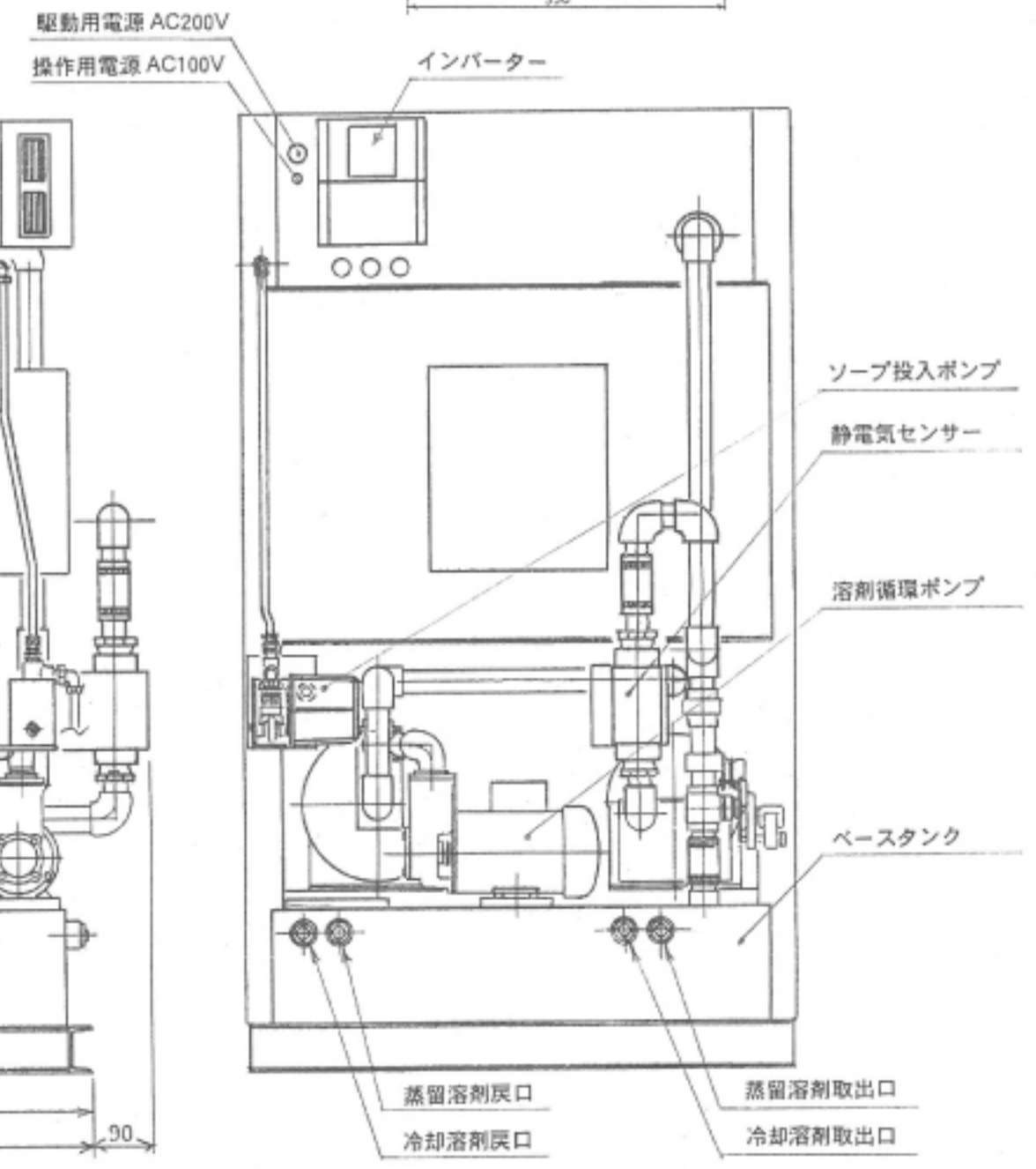
DO100FD 外観図
