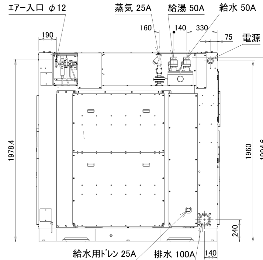
WN1002Z外観図
