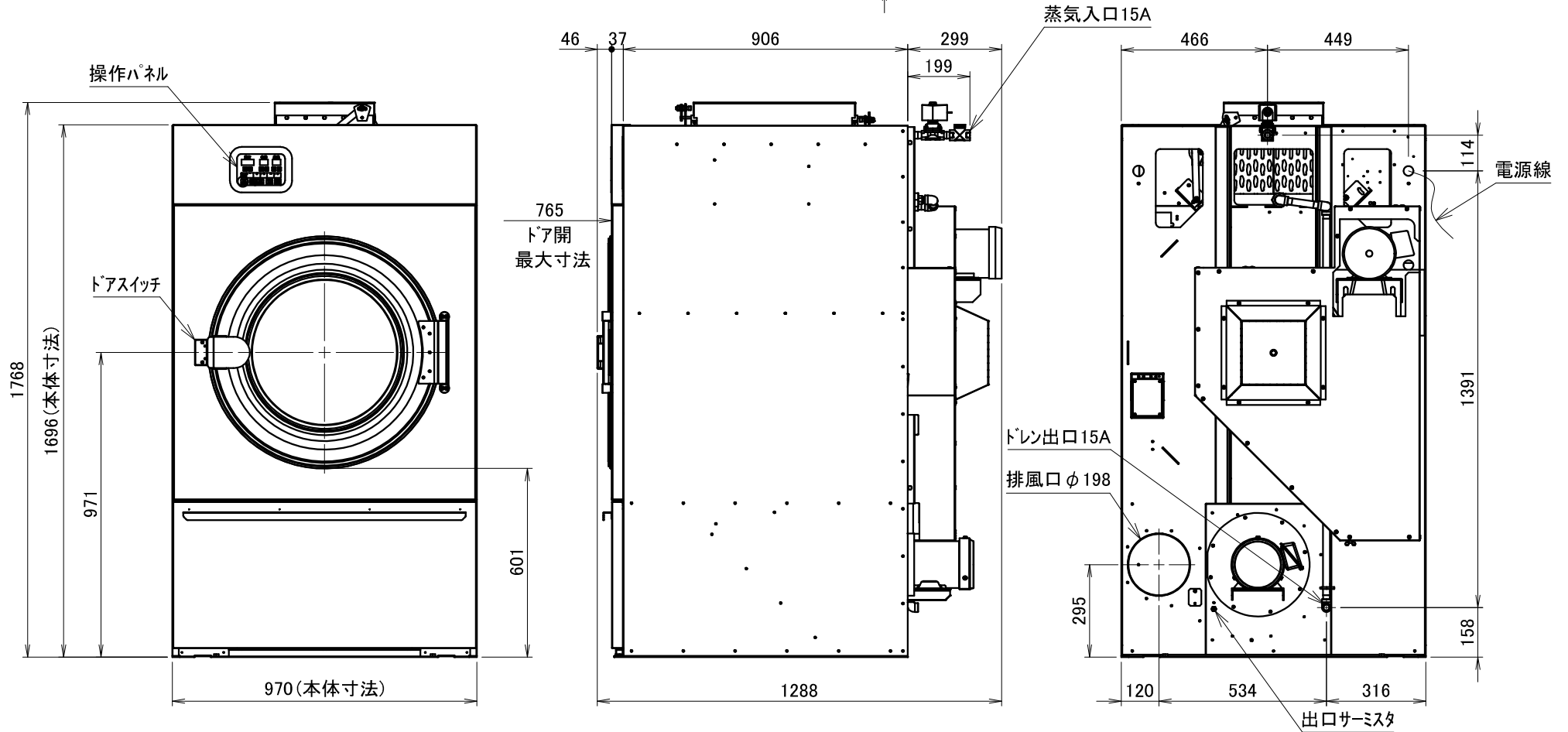
VS262外観図
