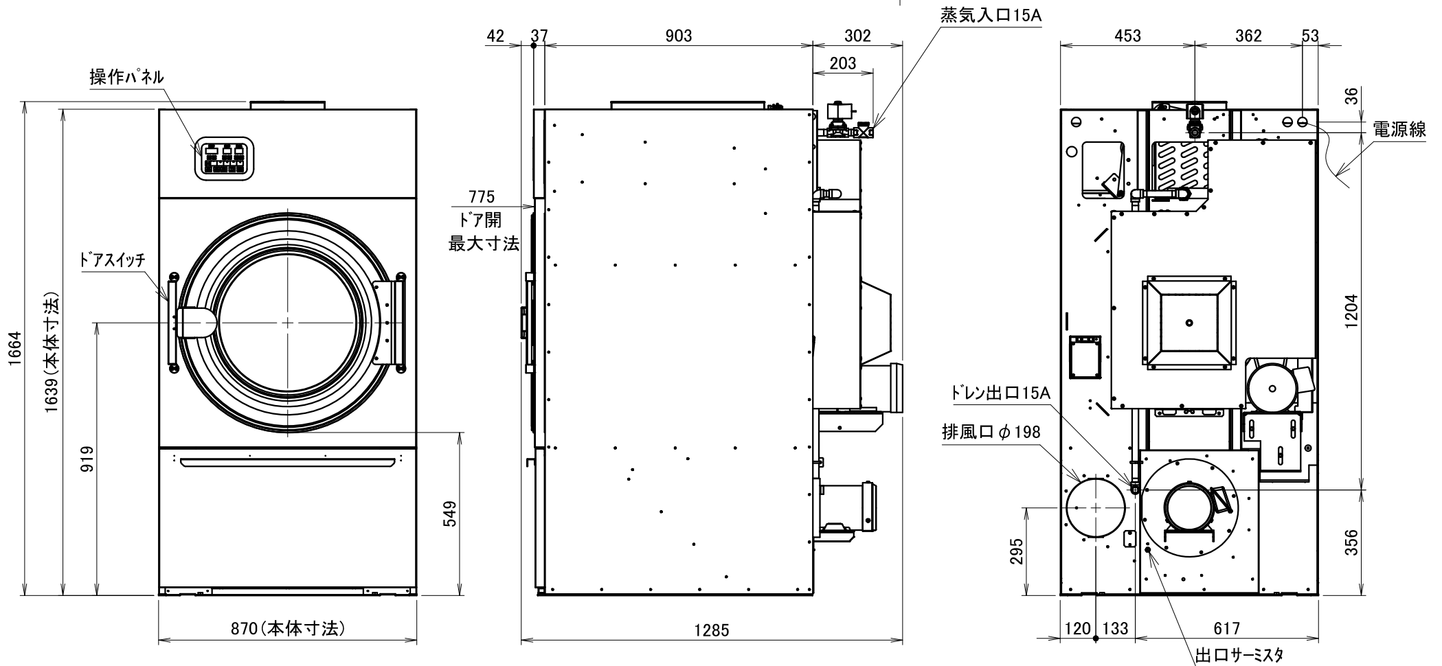
VS201外観図
