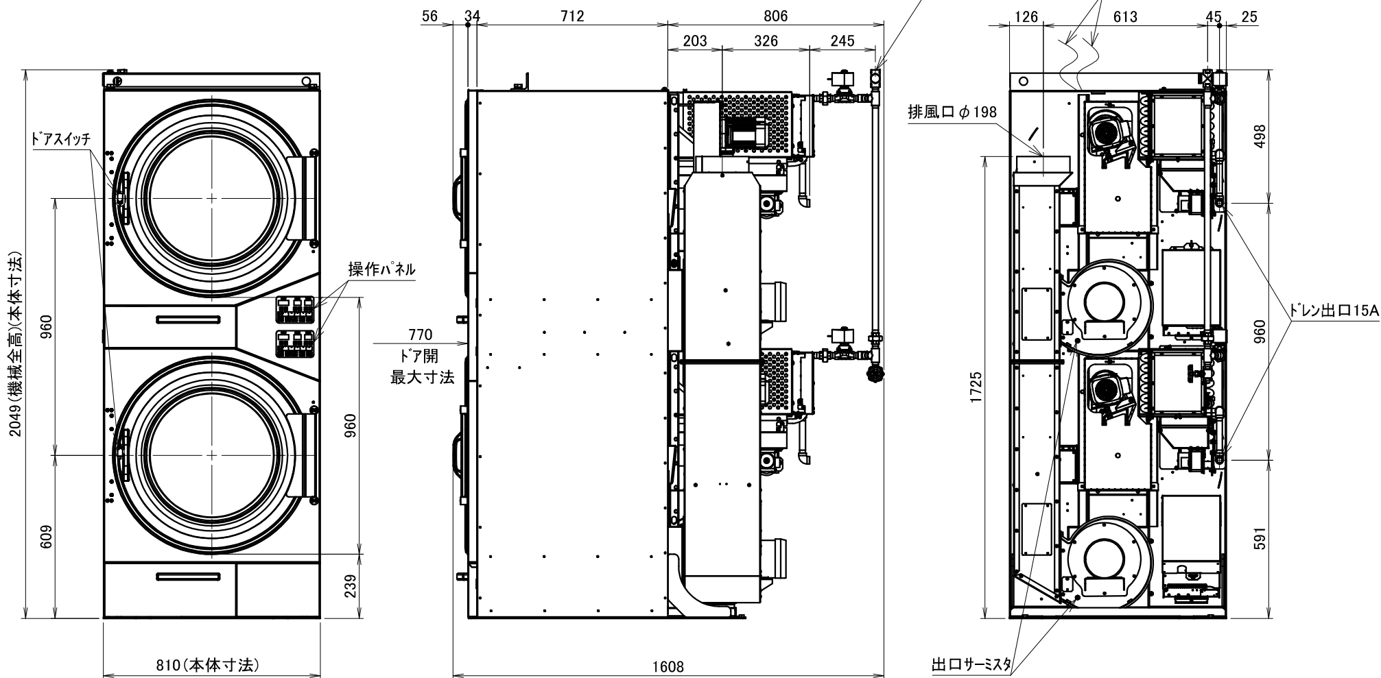
VS133W外観図
