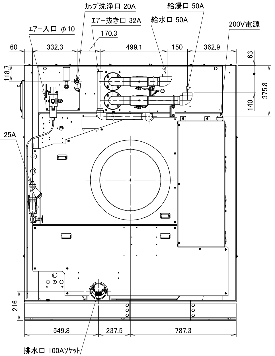
WN630 外観図
