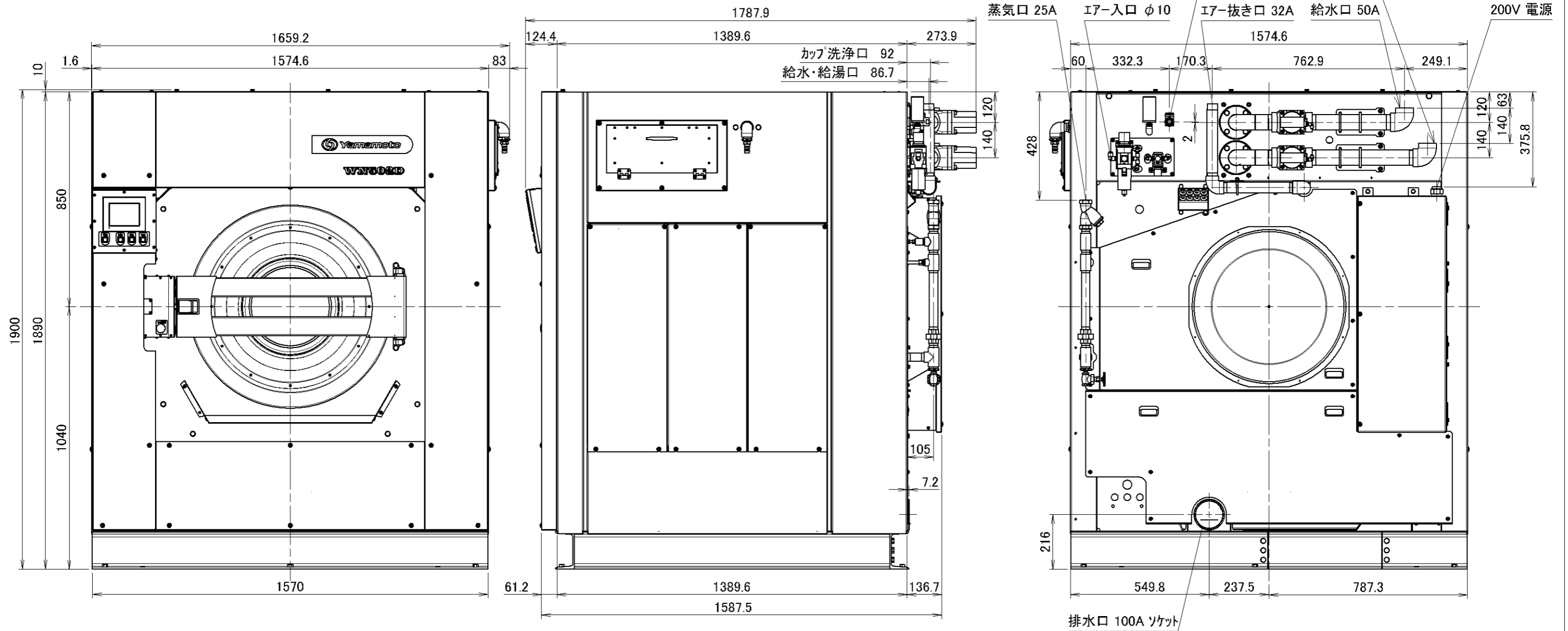
WN502D 外観図
