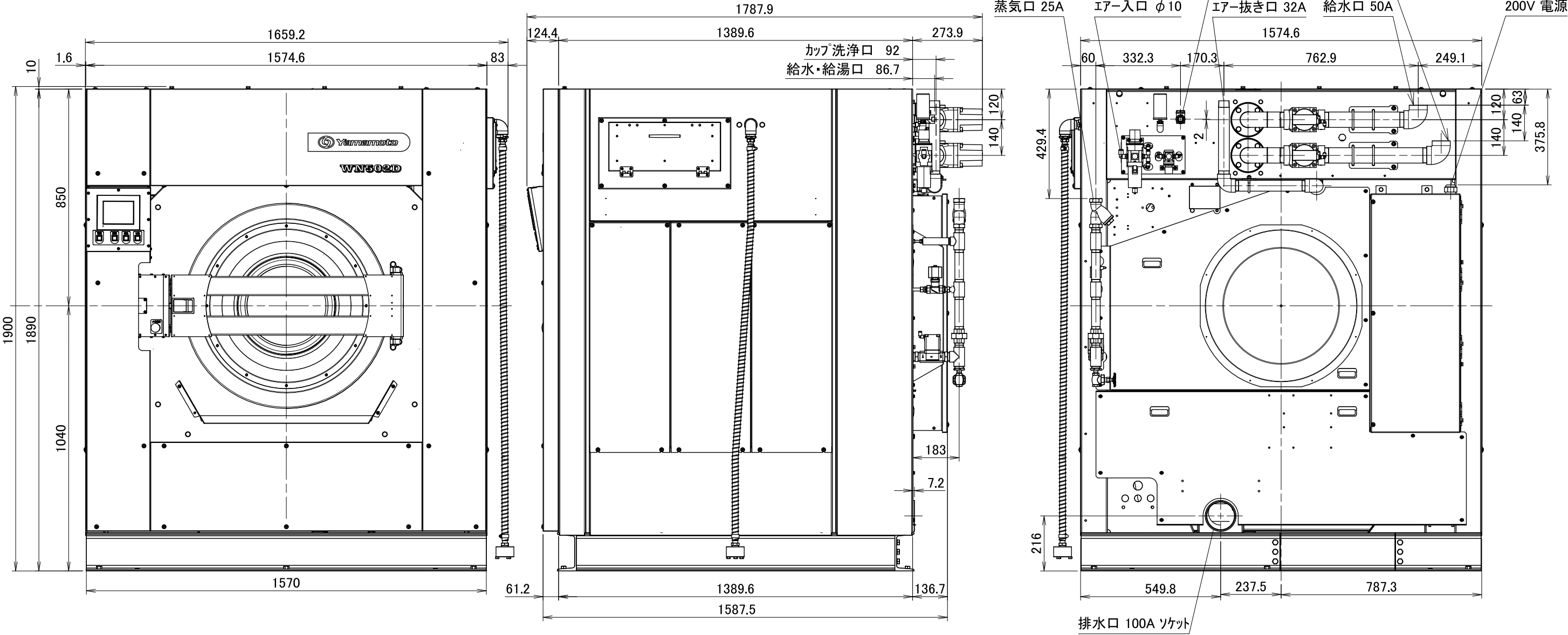
WN502D 外観図
