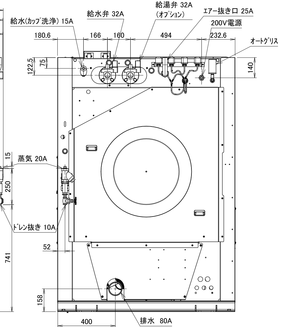
WN430外観図
