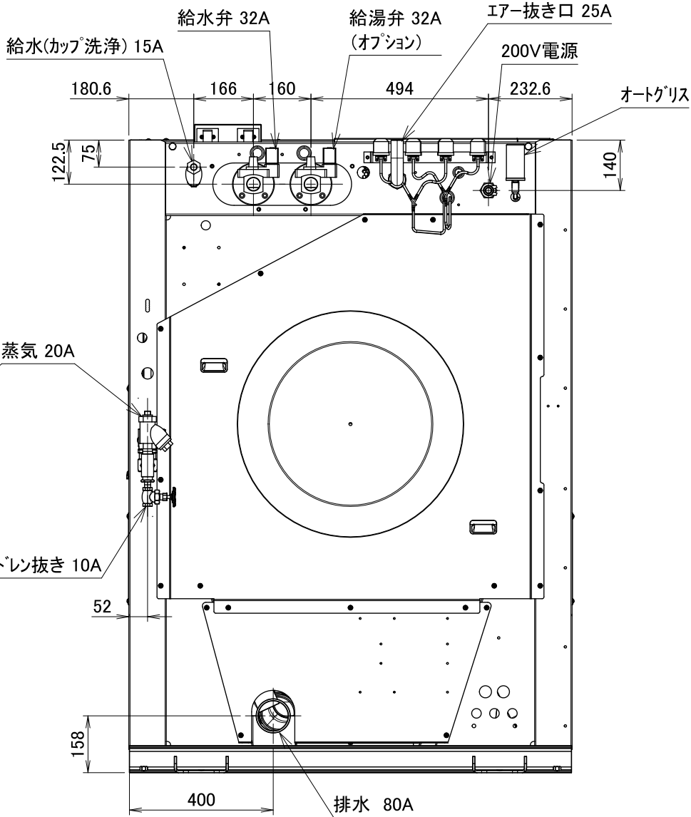
WN360外観図
