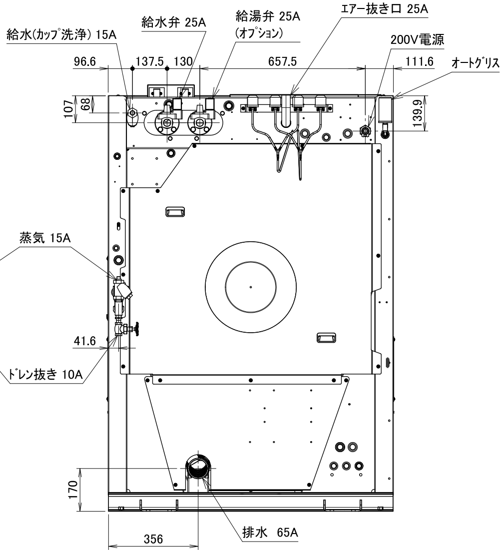
WN280外観図
