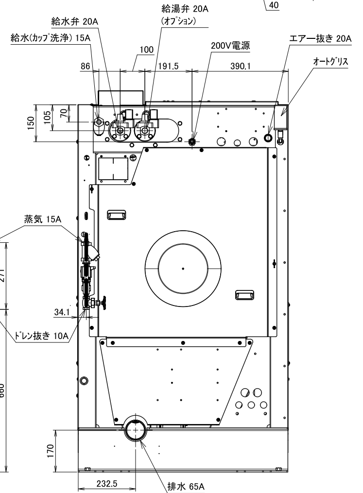
WN130外観図
