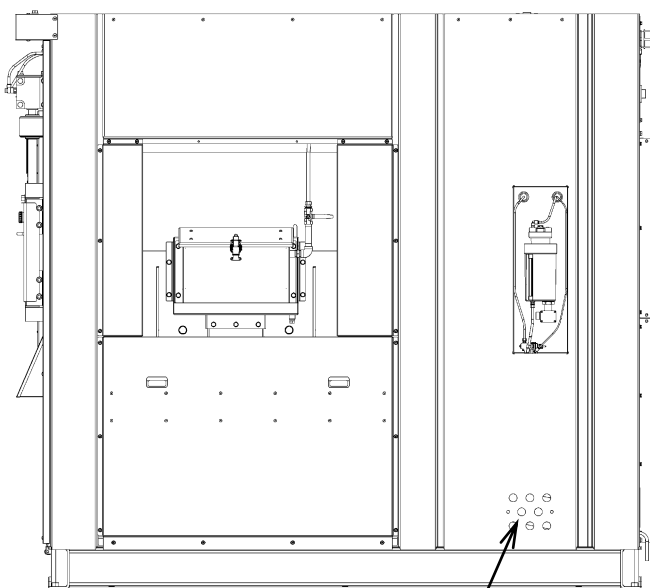
<右側面>
