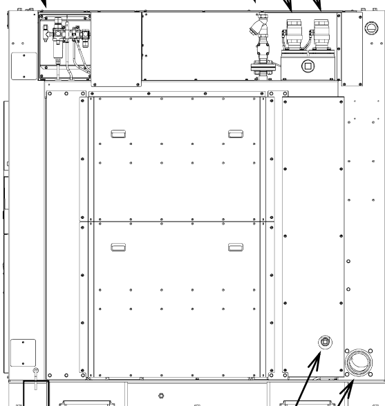
<背面>
