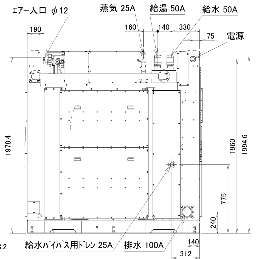
WN1180H外観図
