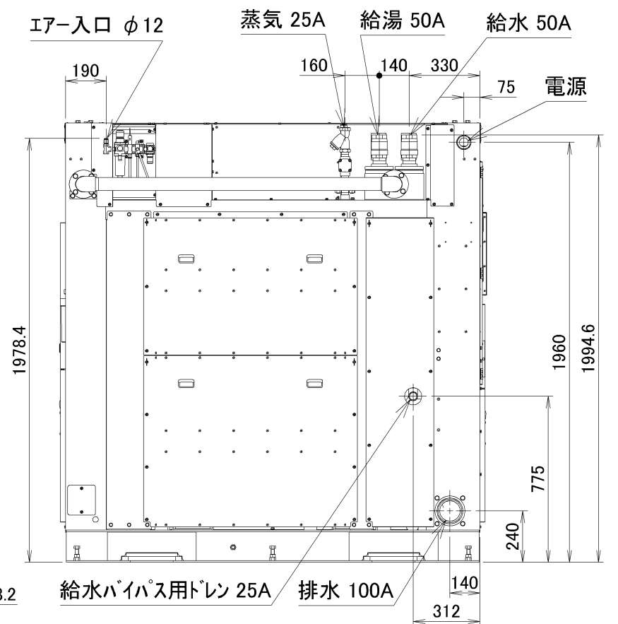
WN1002H外観図
