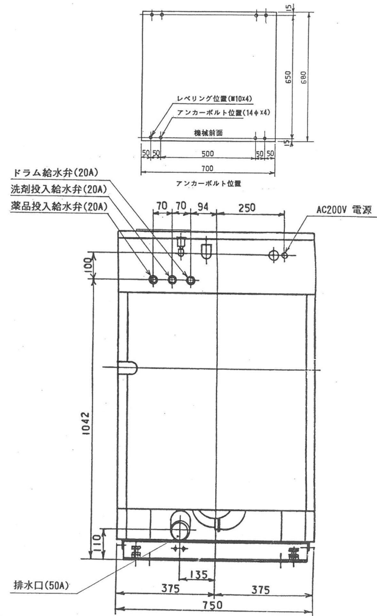
WF90 汚物除去機外観図
