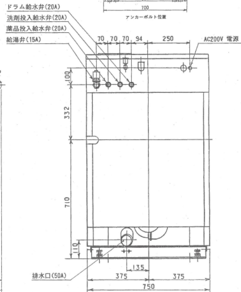
WF90S 汚物除去機外観図（給湯付き蒸気なし）
