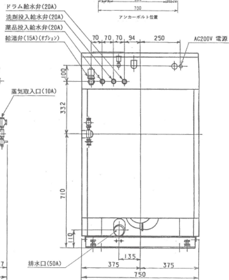
WF90S 汚物除去機外観図(蒸気仕様)
