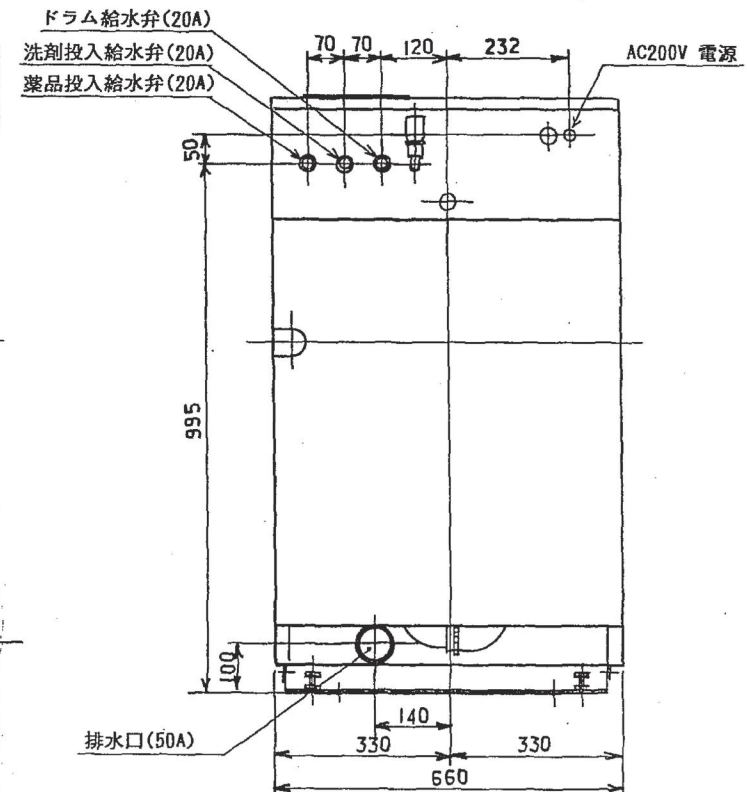
WF90F 汚物除去機外観図 (固定式)
