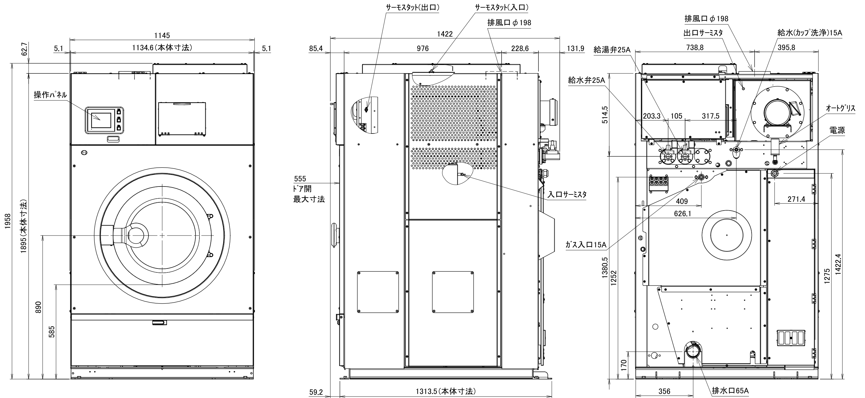
WD352G外觀圖
