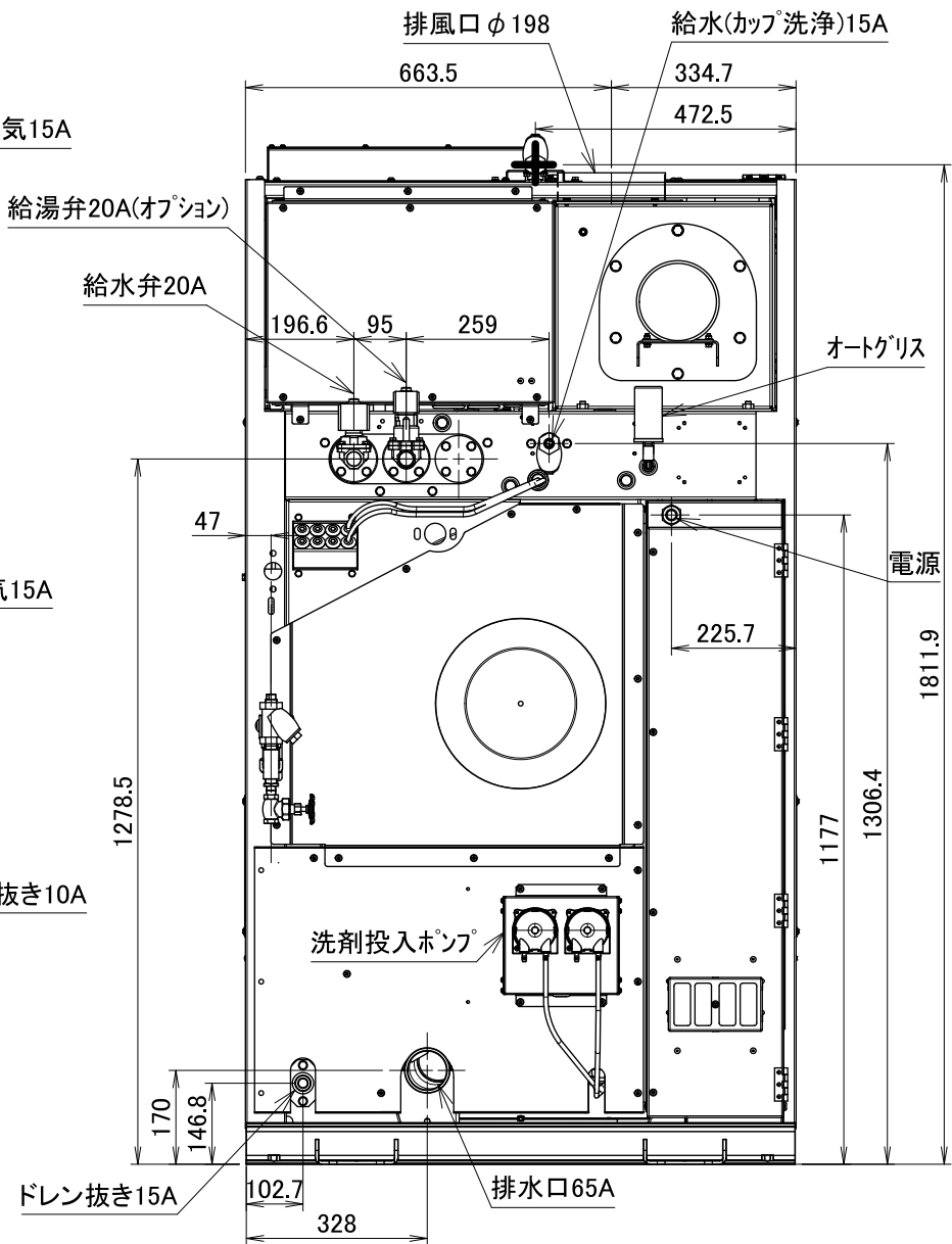
WD272S外観図
