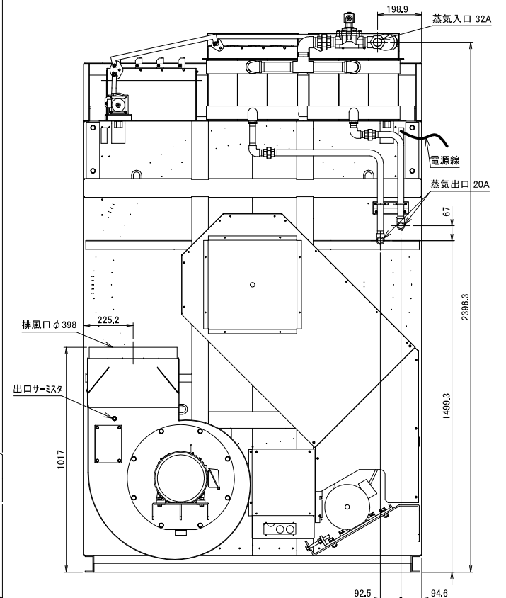
VS723D外観図
