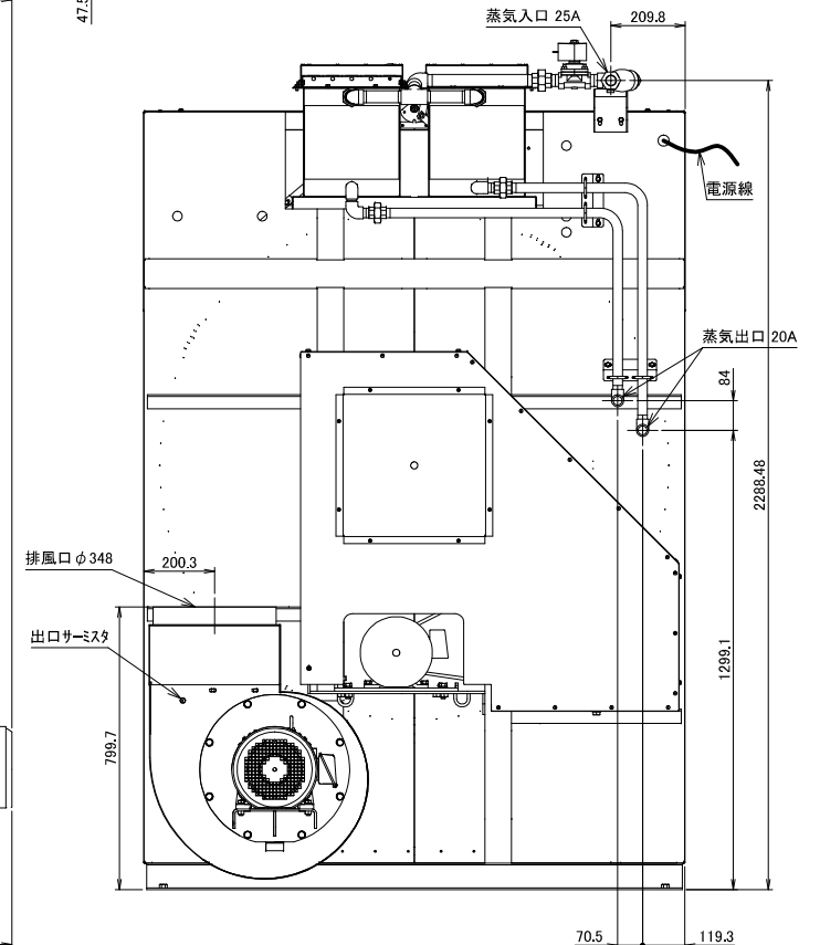
VS723外観図
