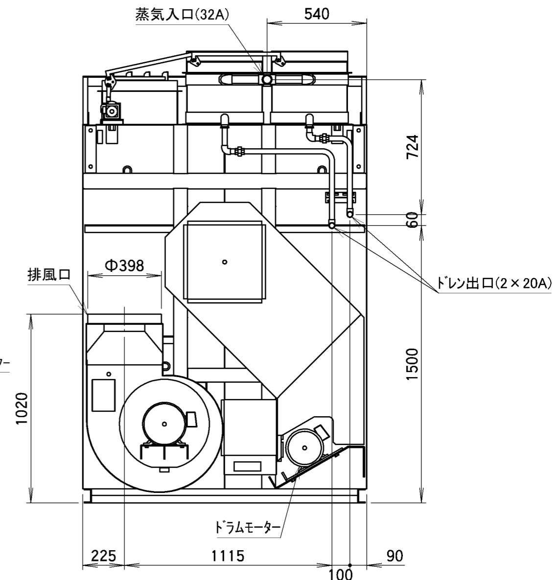
VS500D 外観図
