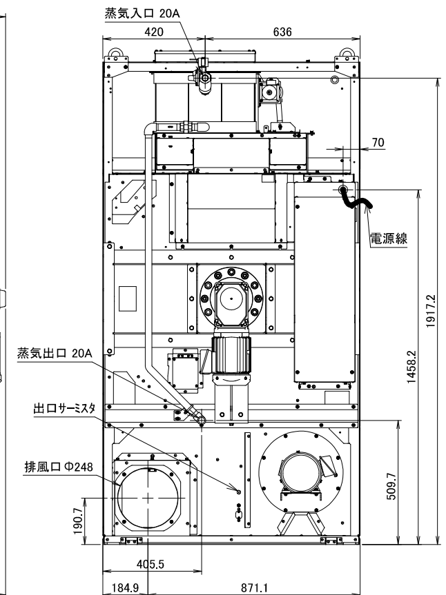
VS383外観図
