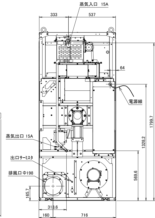
VS253外観図
