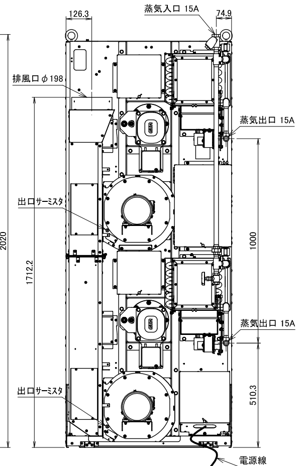
VS143W外観図
