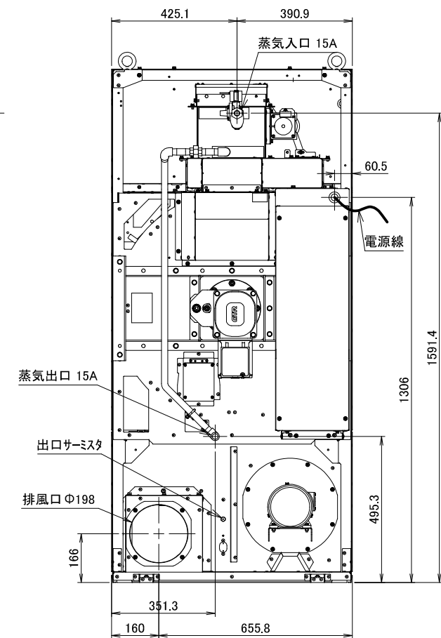
VS143外観図
