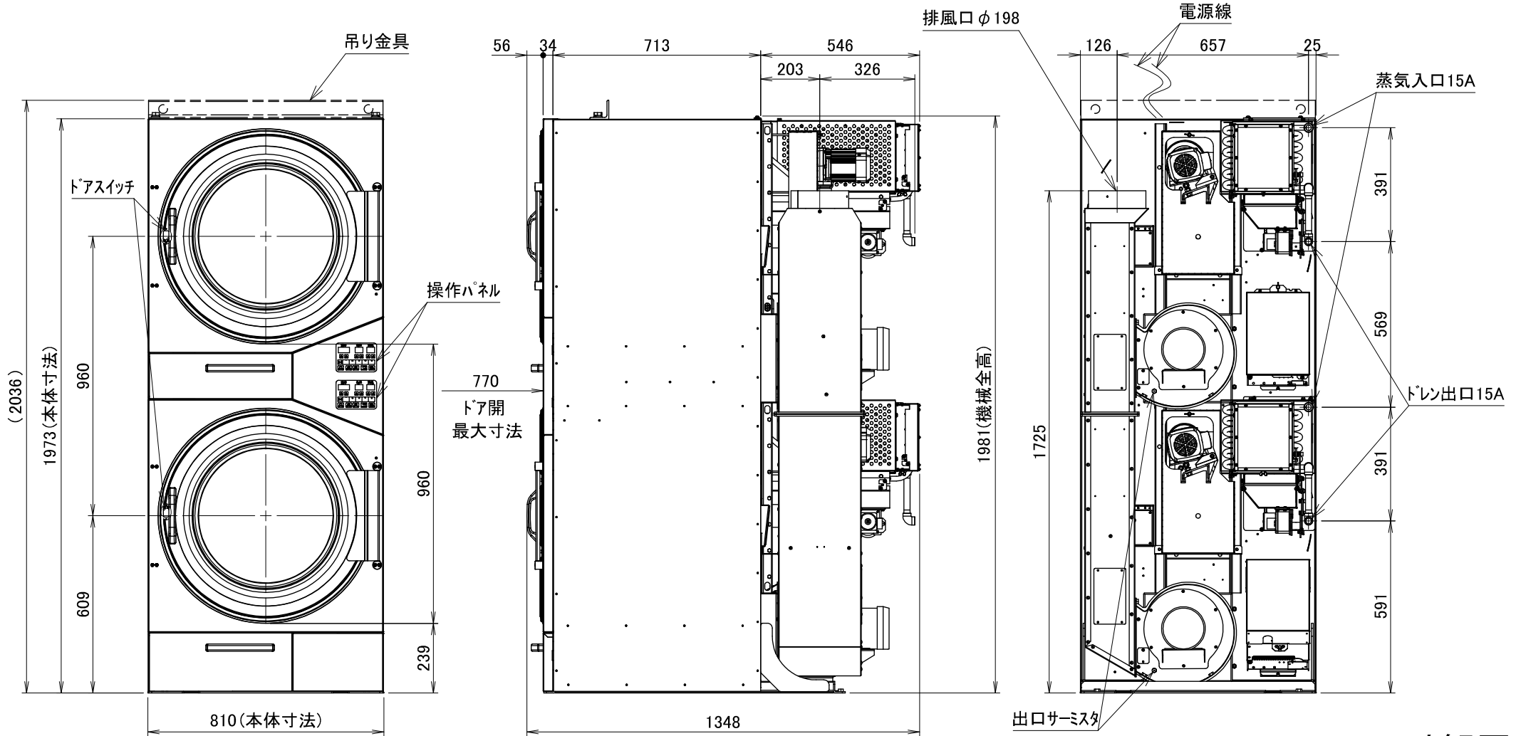
VS111W外観図
