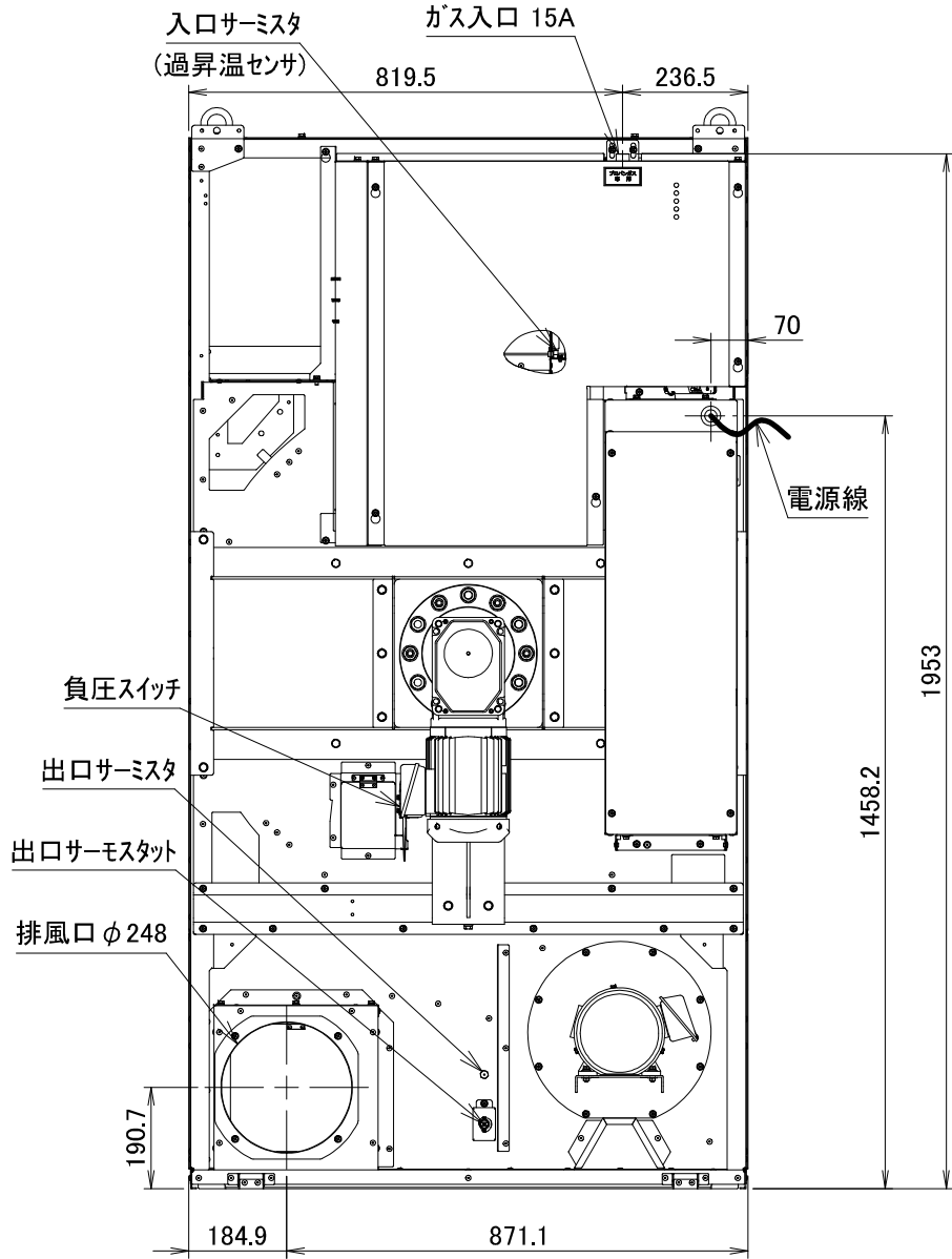
VG383外観図
