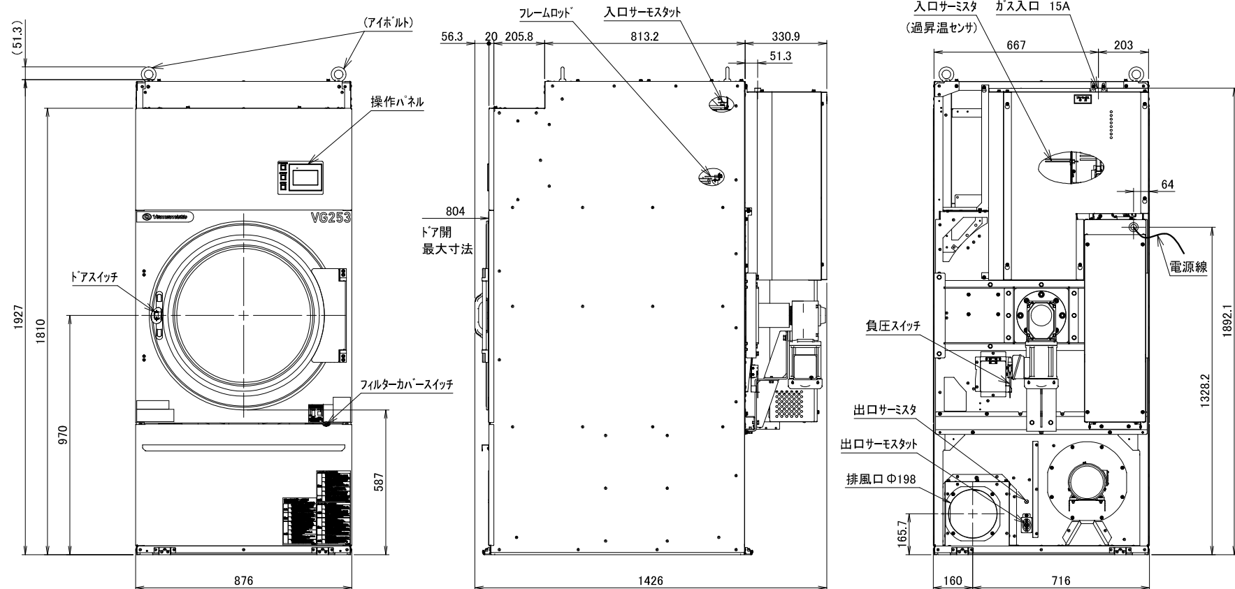
VG253外觀図
