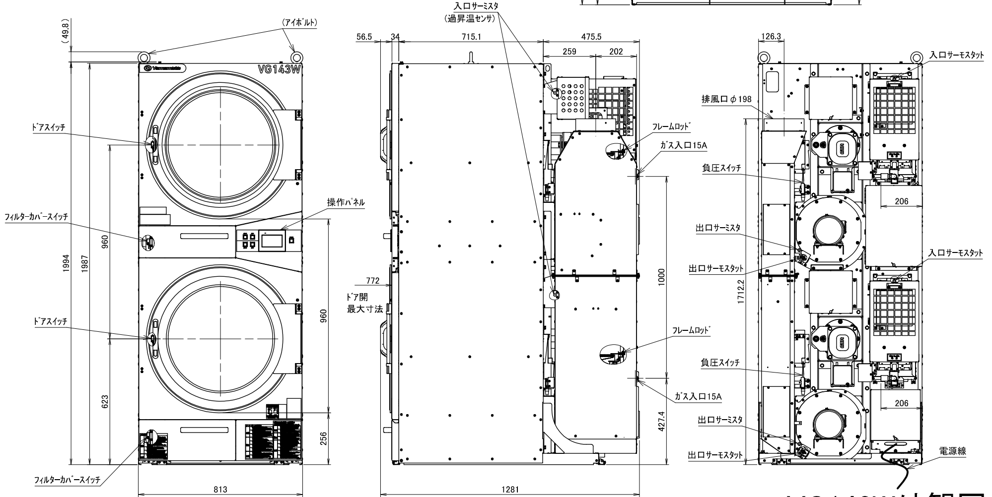
VG143W外観図
