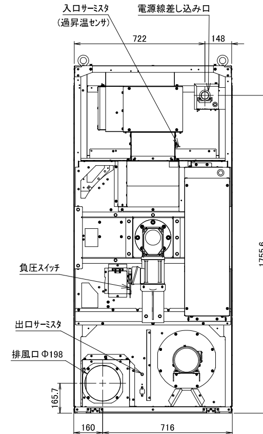
VE253外観図
