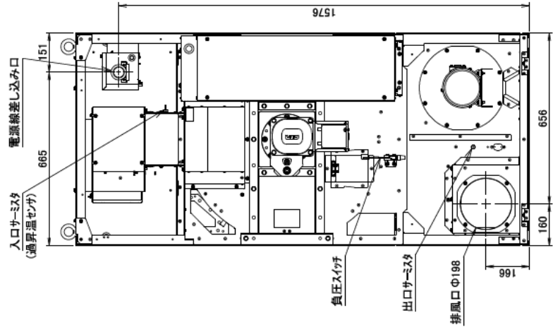
VE143外觀図
