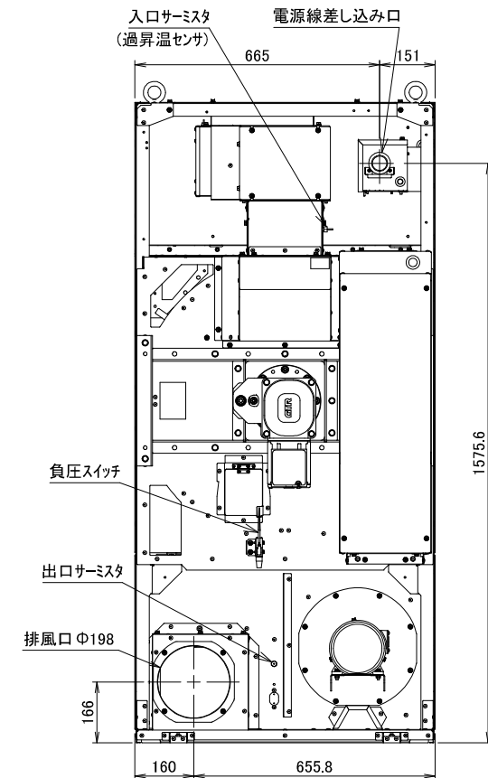
VE143外観図
