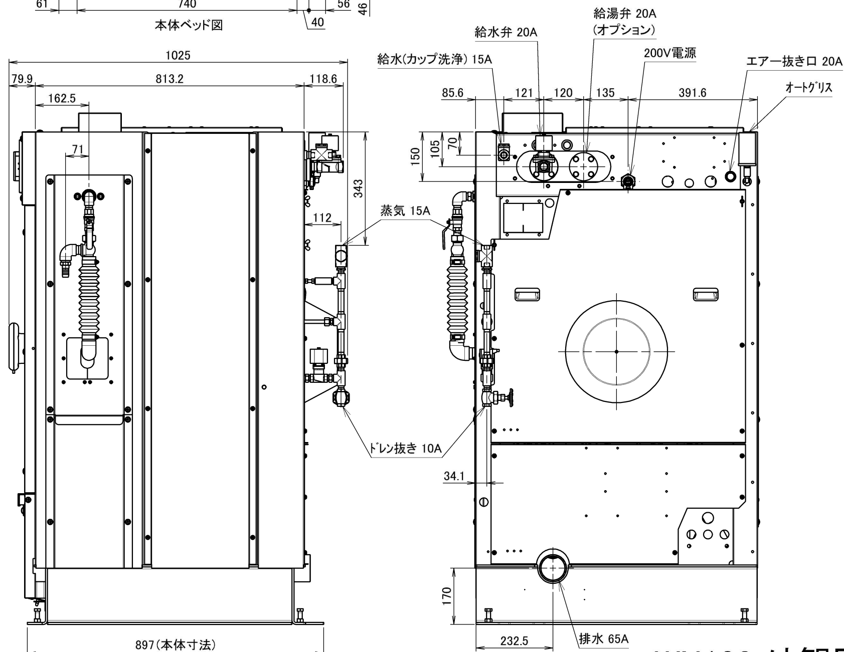
WN103 外観図
