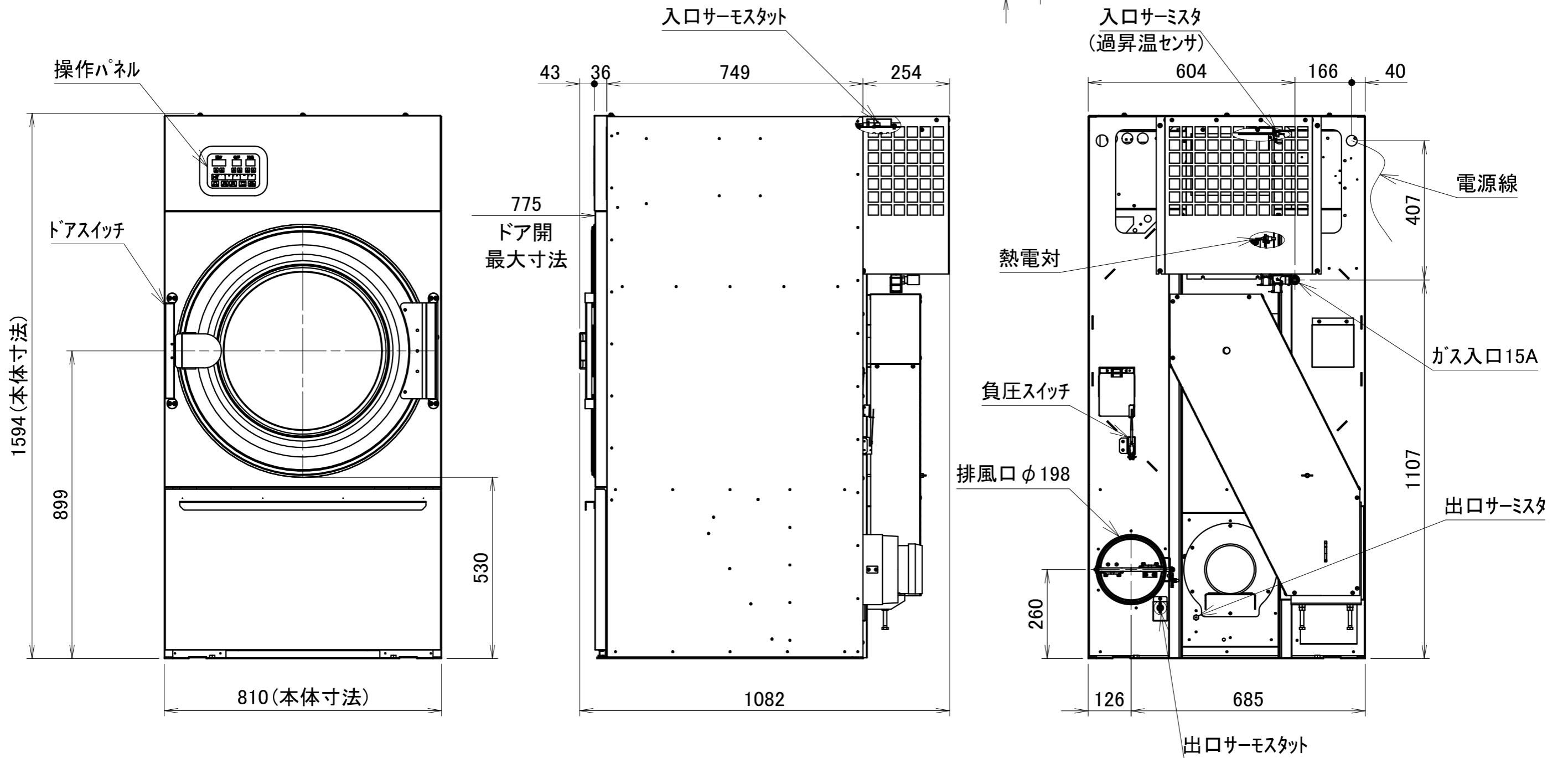
VG132外観図
