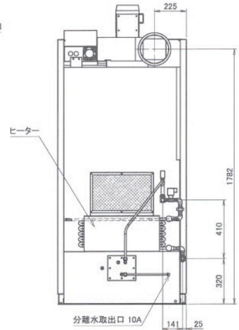
VC1021 外観図
