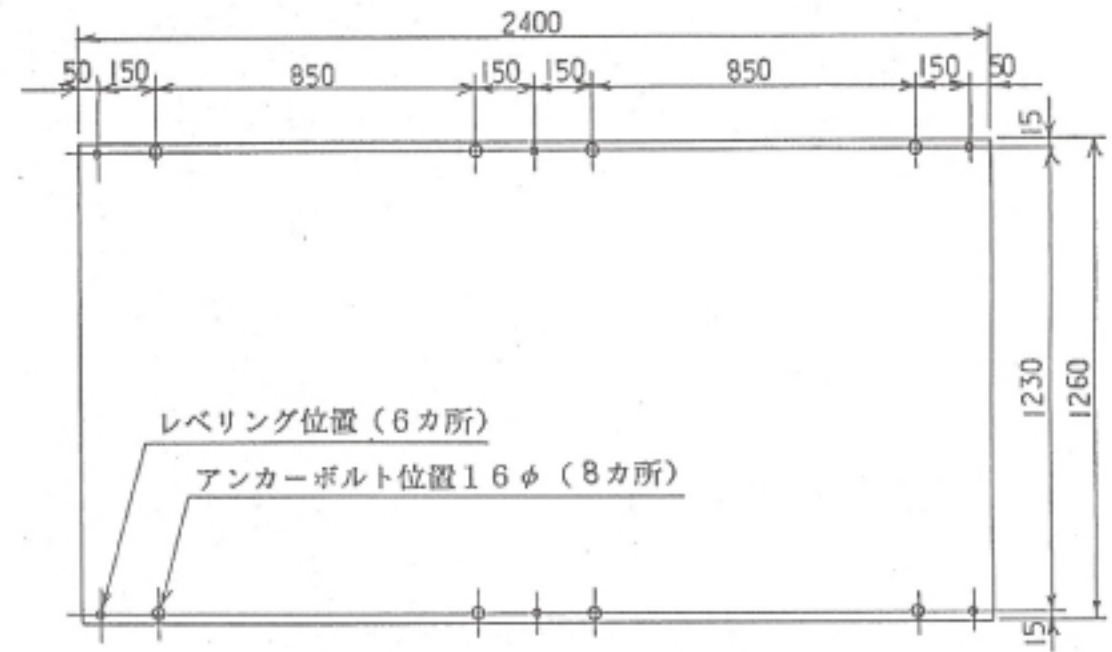
アンカーボルト位置
