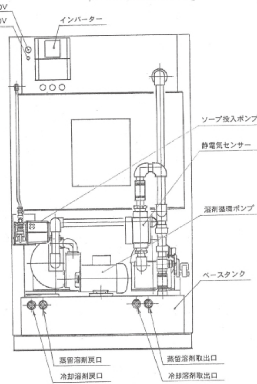
DO100FL 外観図
