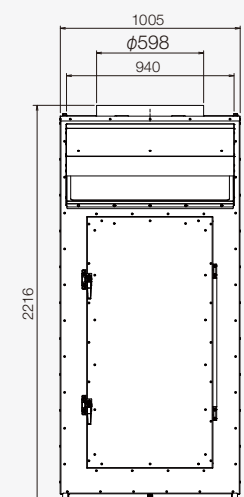
オプション 換気フード付き組立図
