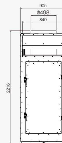
オプション 換気フード付き組立図
