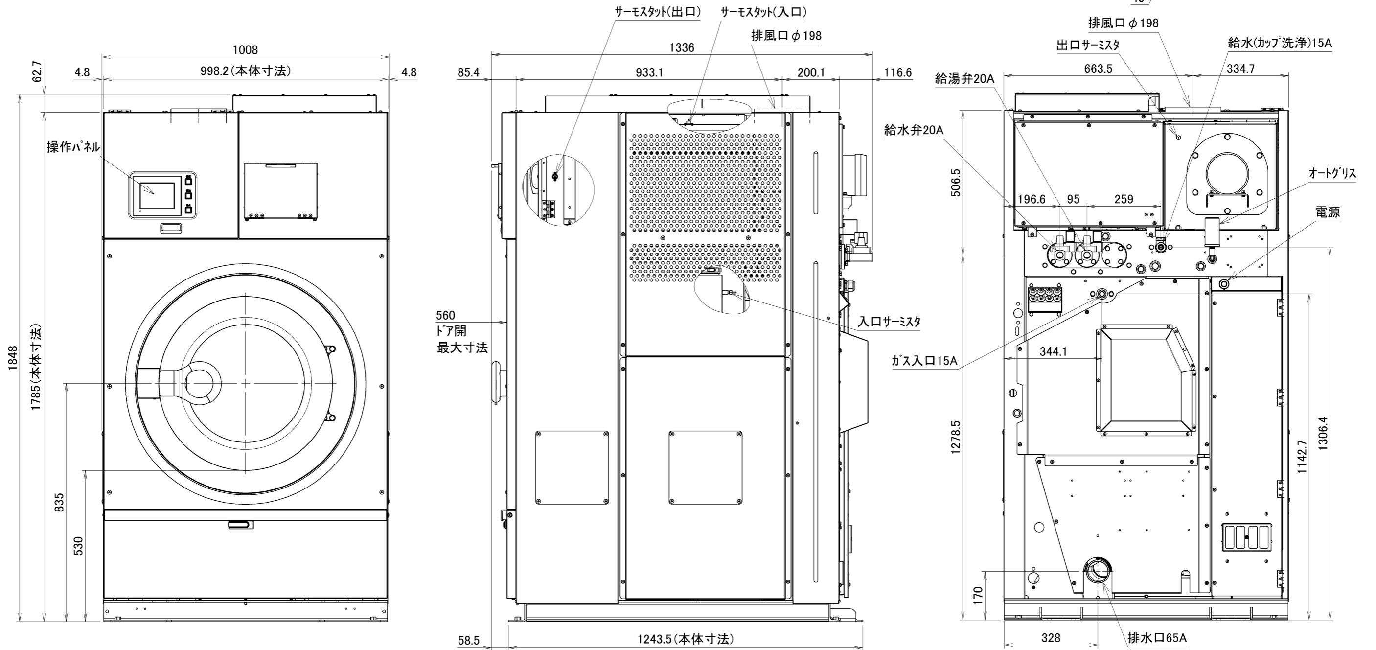
WD252G外観図
