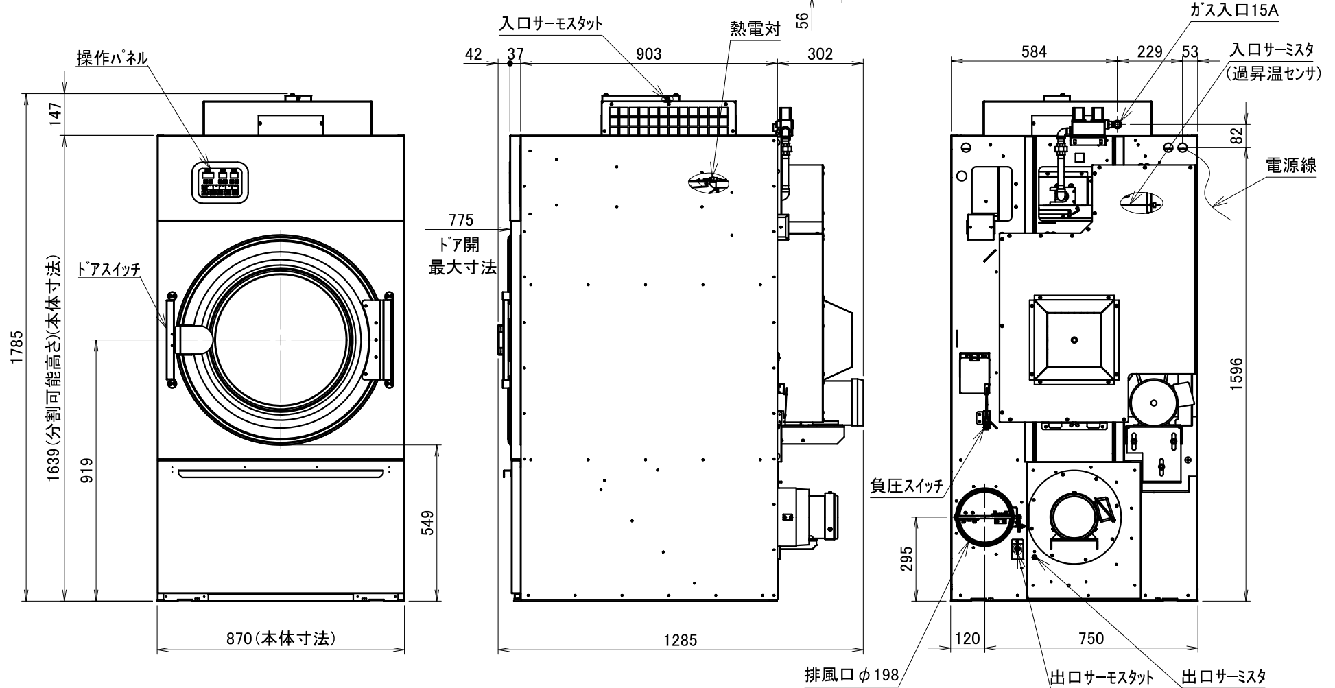
VG201外観図
